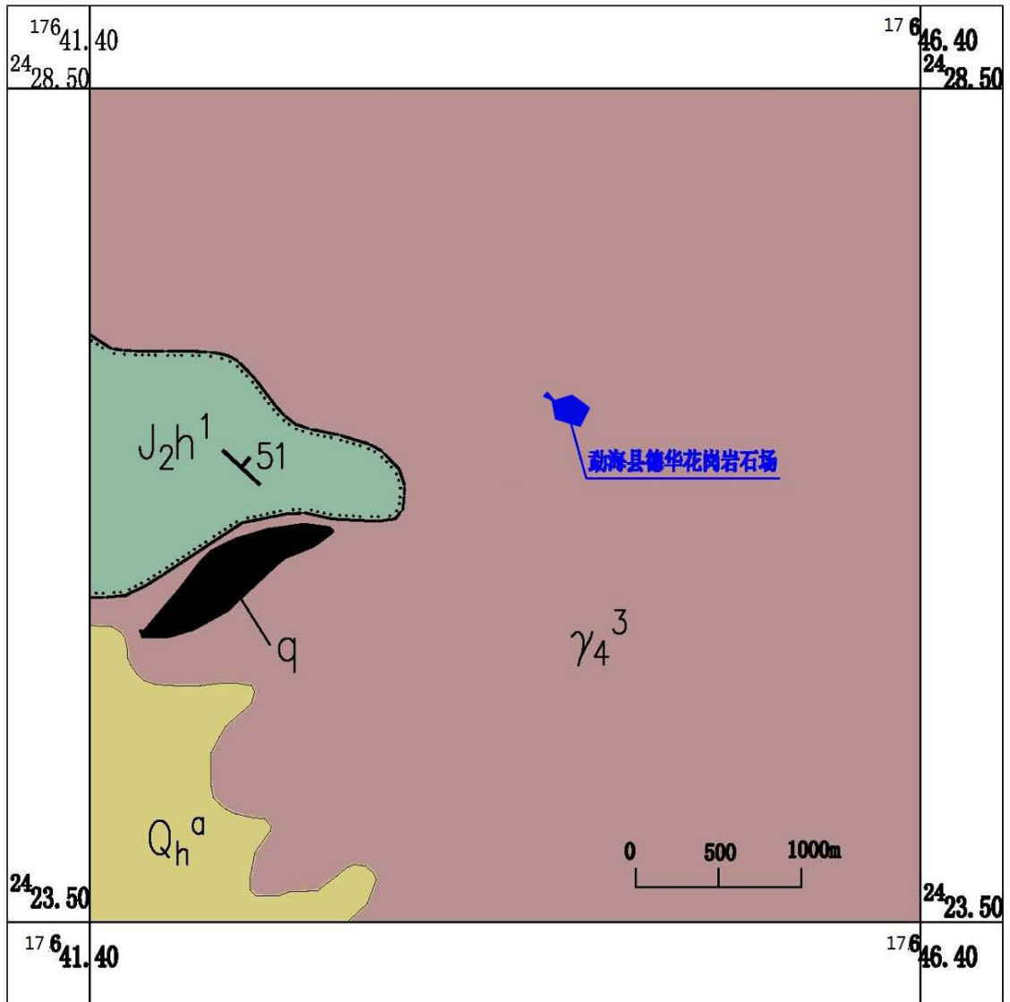
图 3-1 区域地质图
