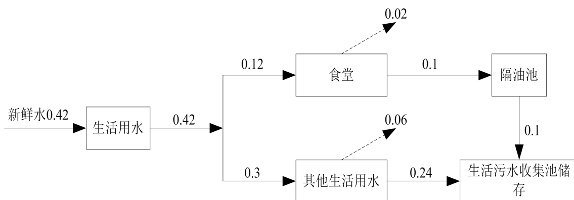
图 5-3 项目区雨天水平衡图 m 3 /d
