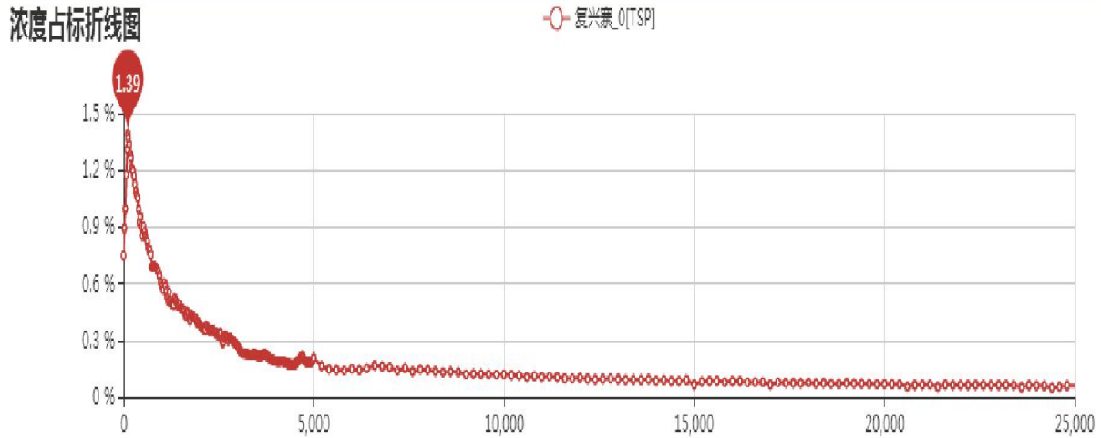
图 7-1 项目无组织排放的颗粒物最大落地浓度及占标率图
