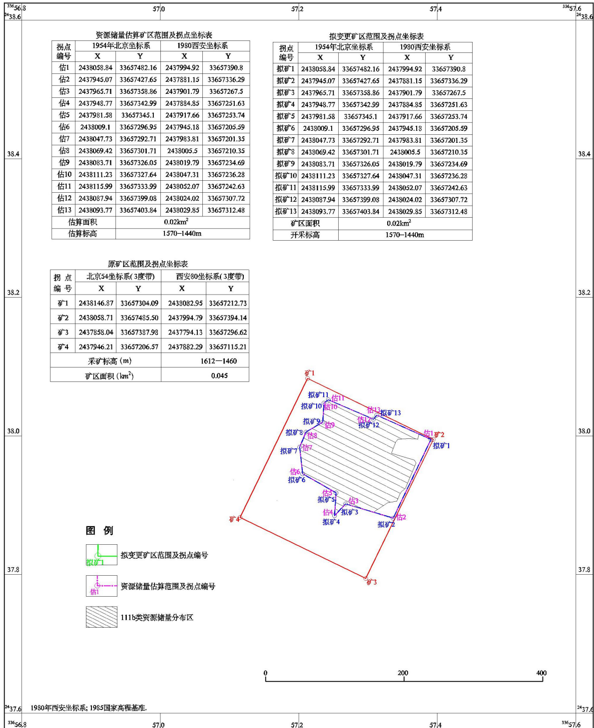
图 1-1 矿界关系图
