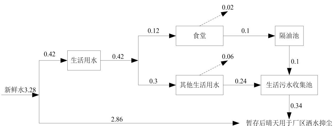
图 5-4 项目区非雨天水平衡图 m 3 /d
