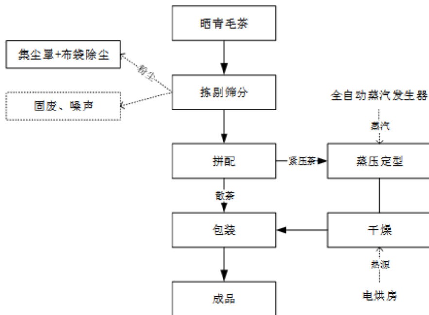
图 5-2 生茶生产工艺流程及产污工序图
