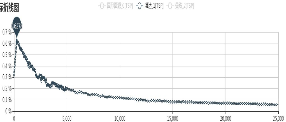
图 7-1 项目无组织排放的颗粒物最大落地浓度及占标率图
