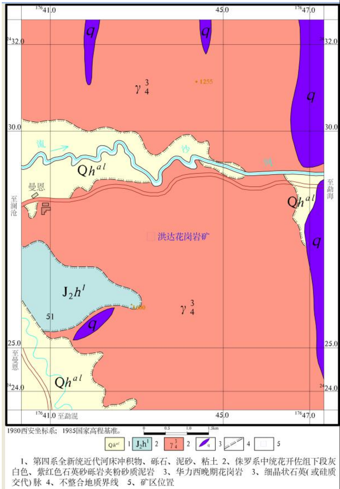
图 2-1 区域地质图
