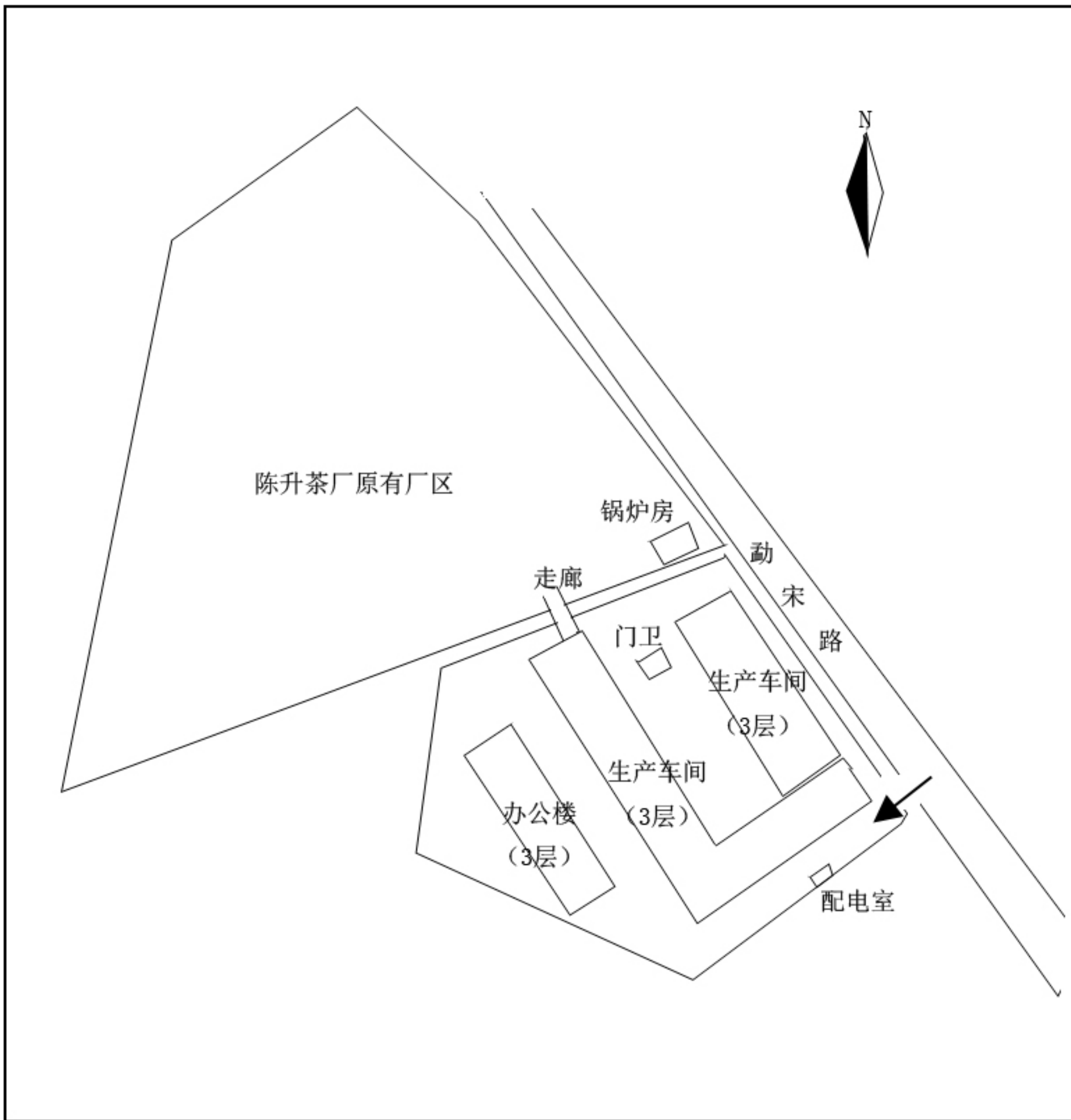
附图3 项目平面布置示意图
