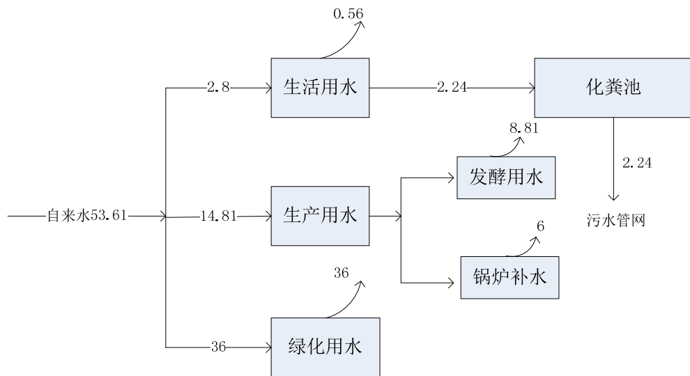
图 5-3 项目水量平衡图 (单位: m 3 /d)
