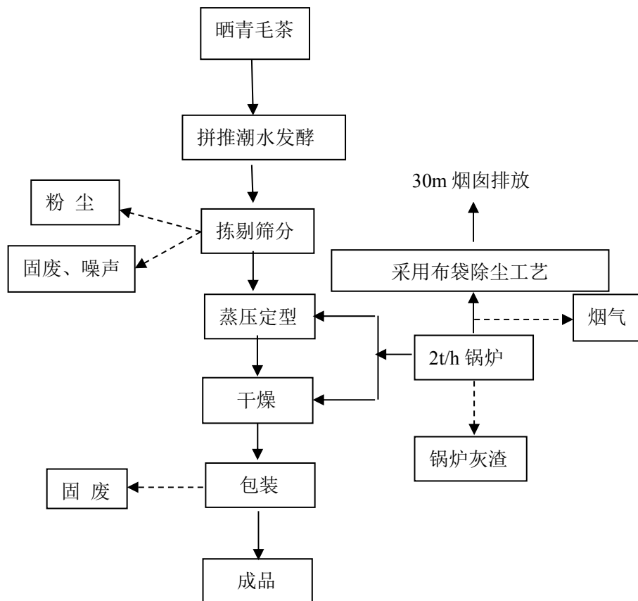
图 5-2 熟茶生产工艺流程及产污工序图
