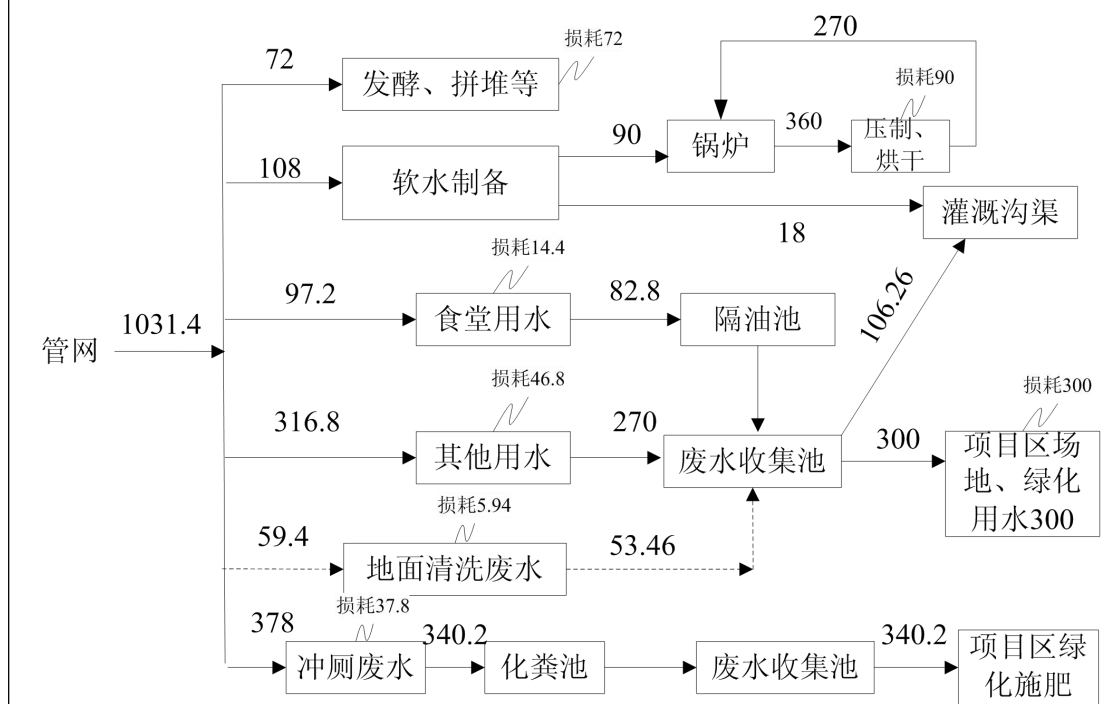
图 5-4 项目全年水平衡图 单位: m³/a
