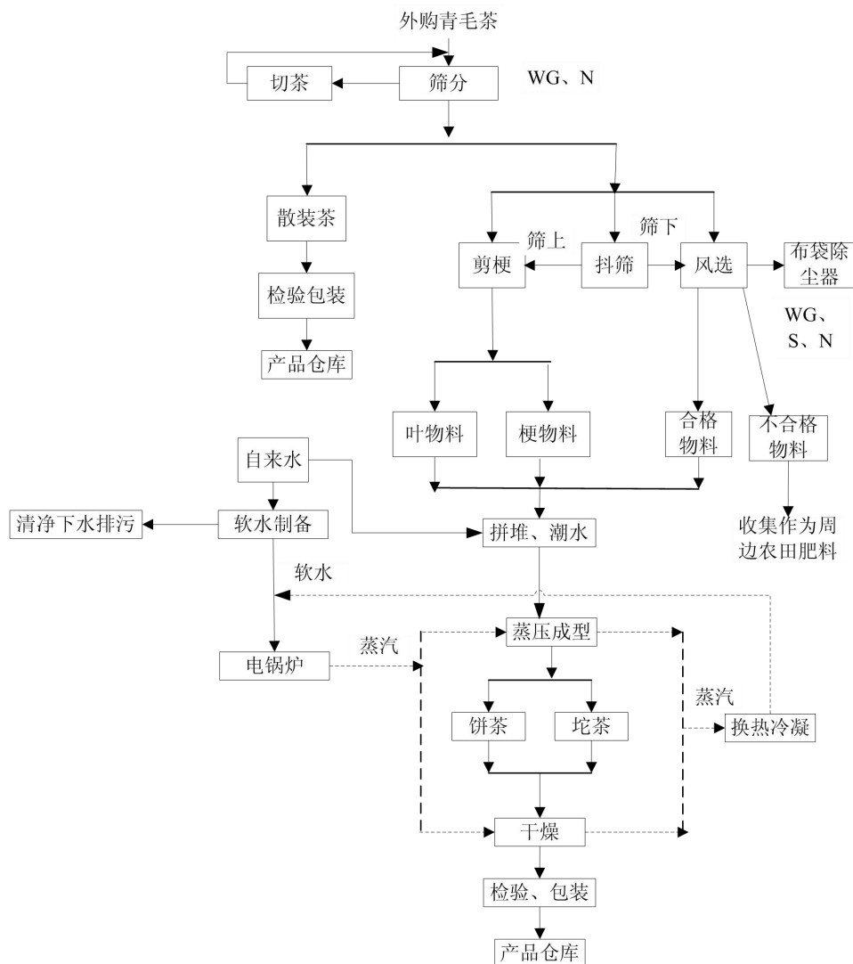
图 5-2 生茶加工、包装工艺流程及污染源图
