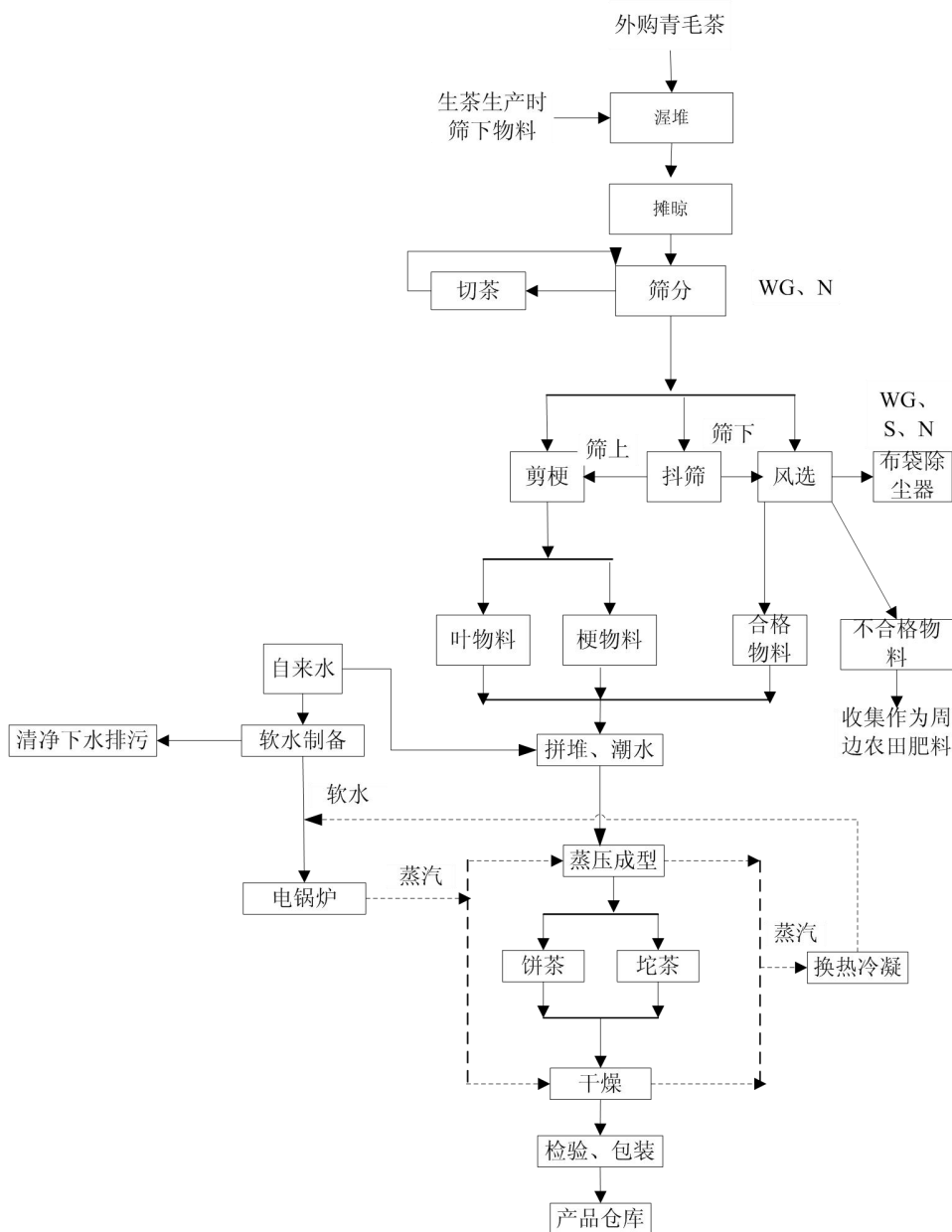
图 5-3 熟茶加工、包装工艺流程及污染源图
