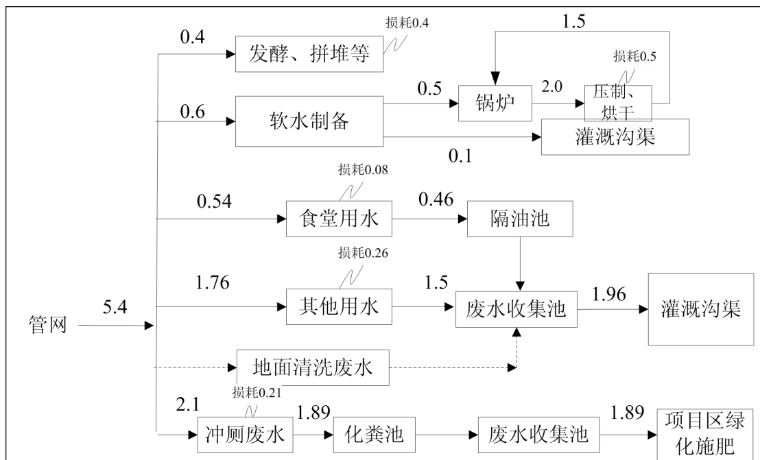
图 5-3 项目雨季水平衡图 单位: m³/d
