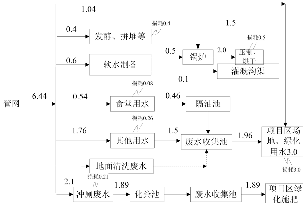
图 5-2 项目旱季水平衡图 单位: m 3 /d
